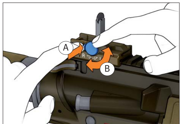
Abb. 36b: Seitenjustierschraube drehen
