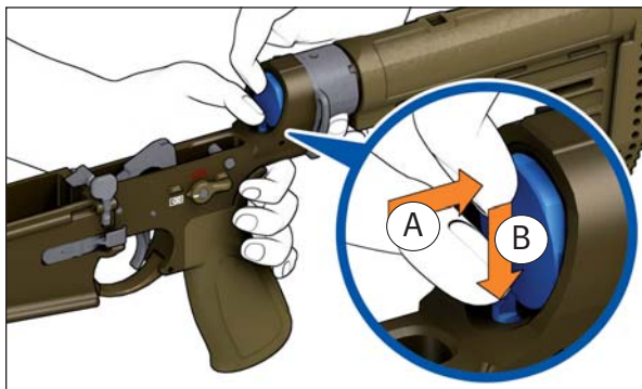
Abb. 50a: Haltebolzen für Puffer eindrücken
