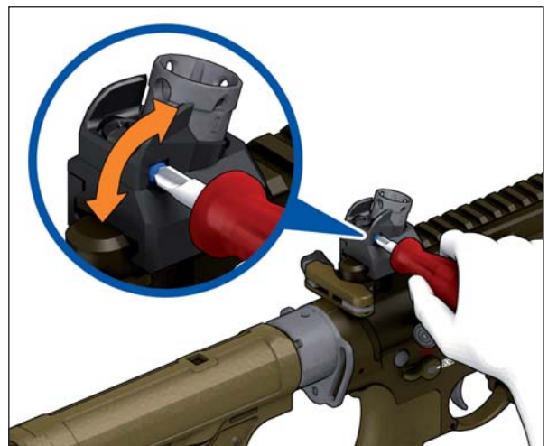
Abb. 35c: Seitenjustierschraube drehen
