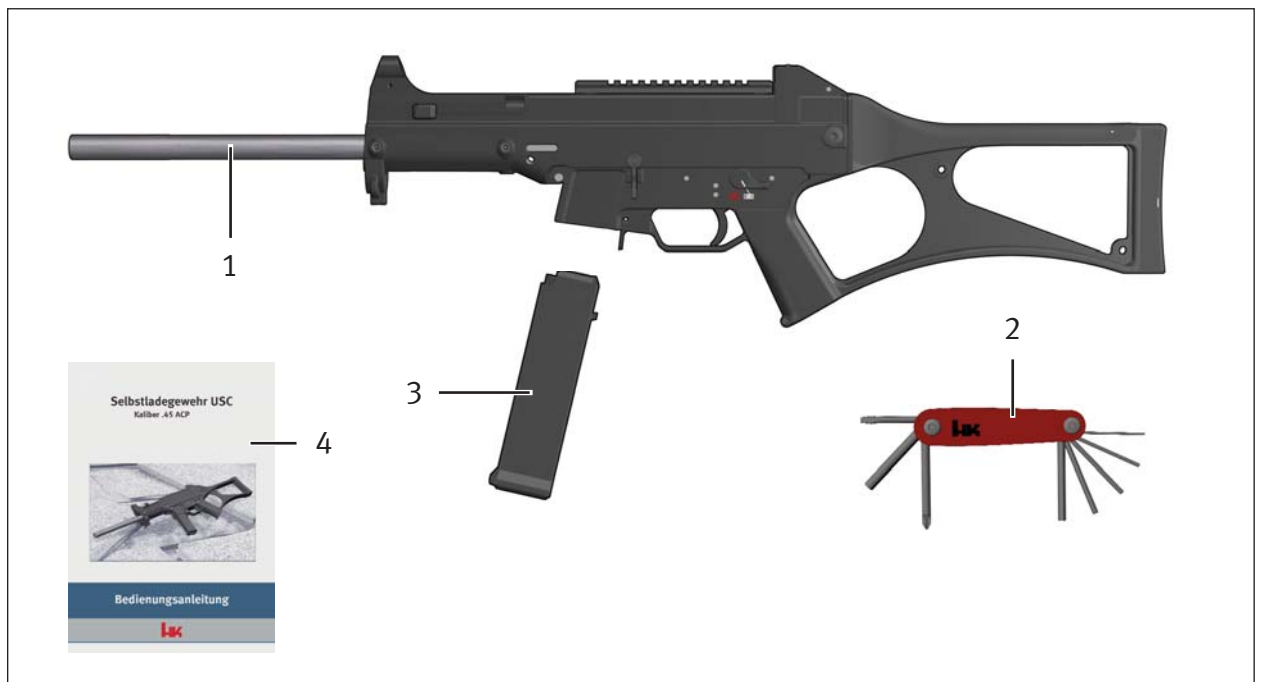
Abb. 10a: Selbstladegewehr USC, Kaliber .45 ACP
