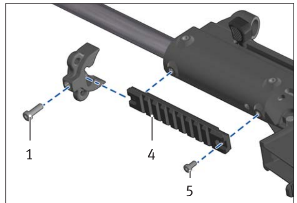
Abb. 27b: Picatinny-Schiene umbauen
